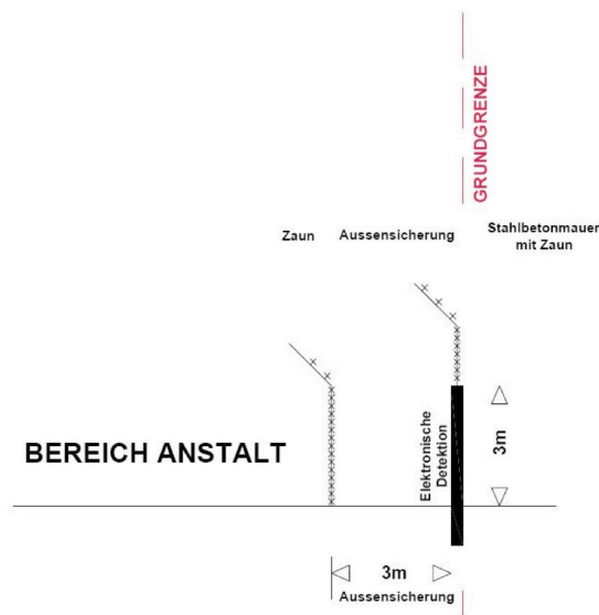
BILDUNTERSCHRIFT Eines technische Skizze des Sicherheitszauns in der Ausschreibung. Foto: http://www.architekturwettbewerb.at/data/media/med_binary/original/1264673999.pdf
